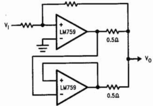
Paralleling LM759 Power Op Amps
